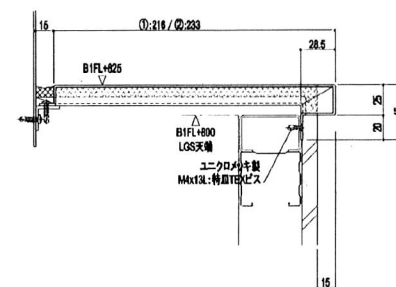
<< 【I】部断面詳細図 >>
