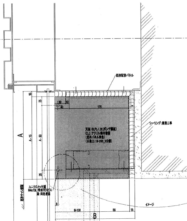
<< 天板③~⑤平面詳細図 >>
