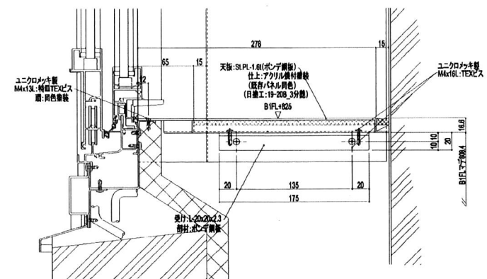
<< 【A】部断面詳細図 >>
