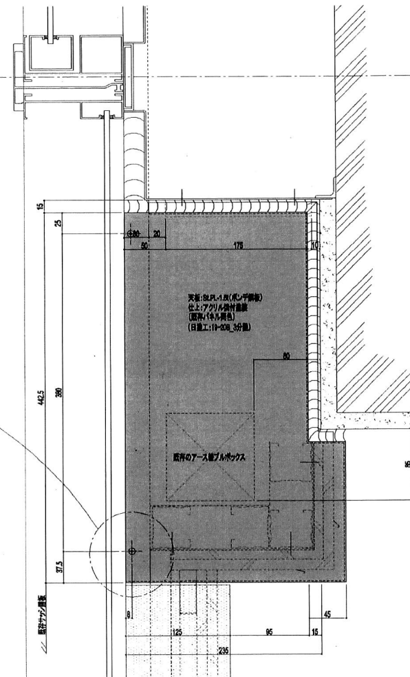
<< 天板⑦平面詳細図 >>
