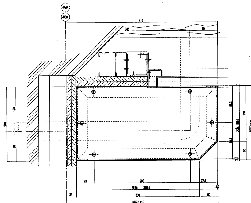
<< 天端平面図 >>
