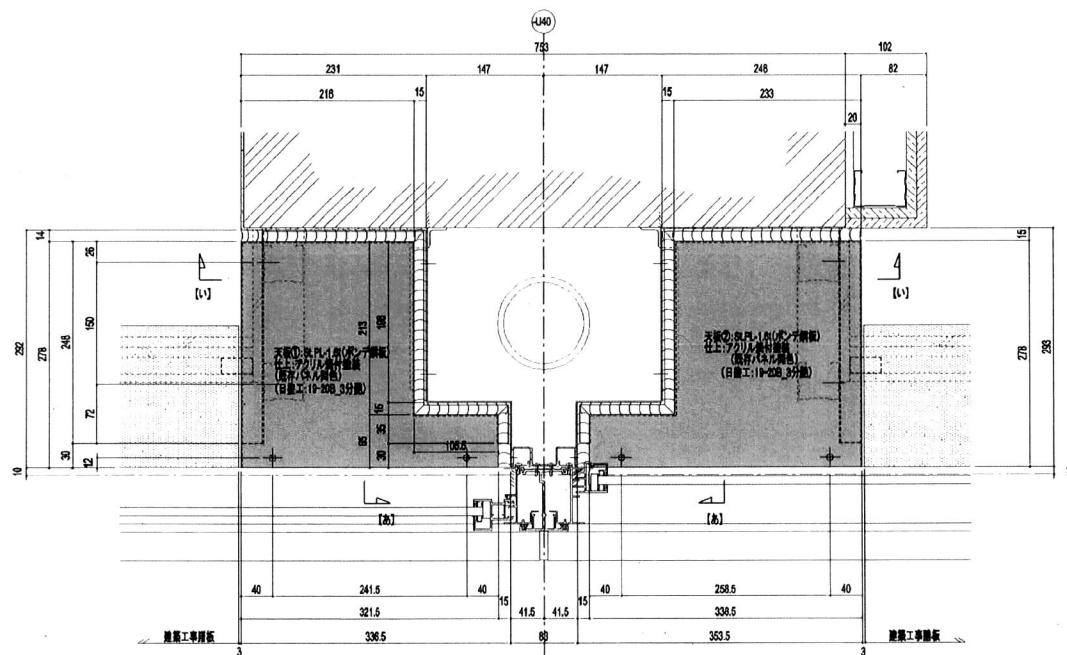
<< 天板①・②平面詳細図 >>
