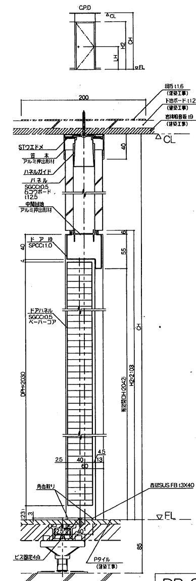
縱断面図
