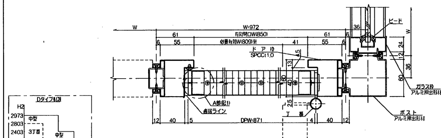
片開き横断面図
