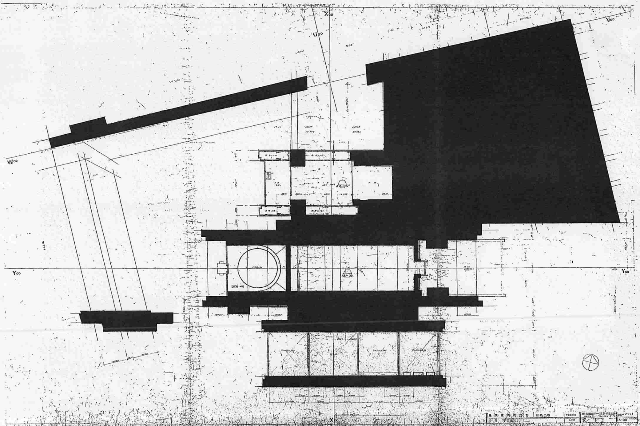
5階平面図
