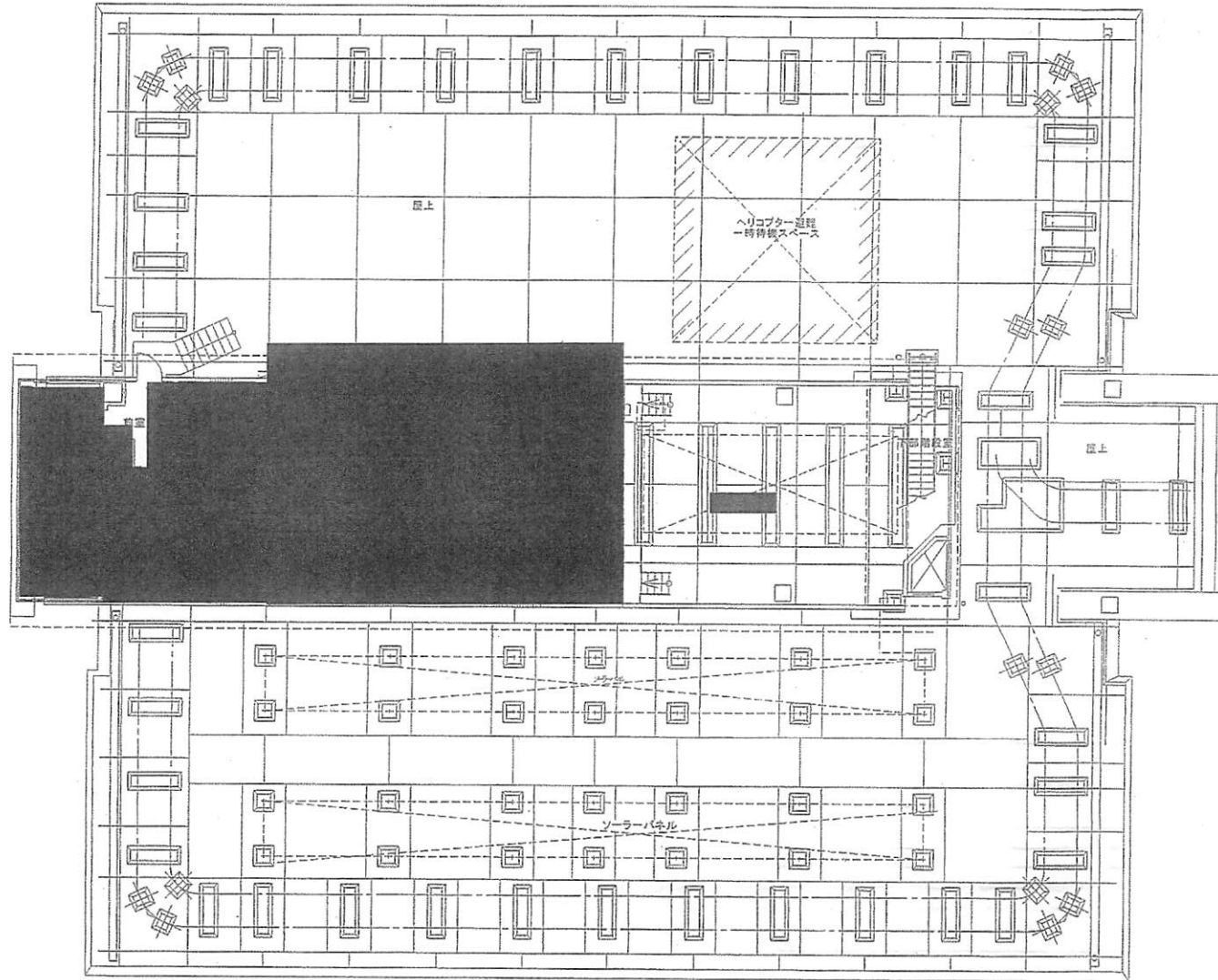
新館 PH階平面図 (S=1/200)
